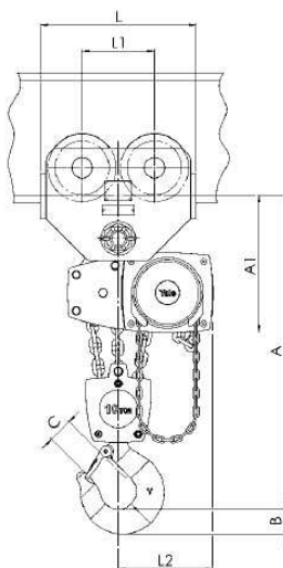
Yalelift ITG, 10.000 kg
