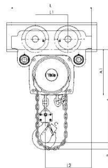
Yalelift ITG, 500 - 3.000 kg
