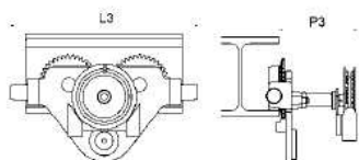
HTP 500 - 5.000 kg s otočným ručním řetězem a gumovými nárazníky
