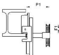
HTG 10.000 kg, ruční zařízení
