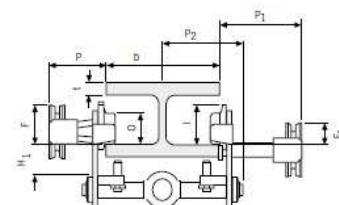
HTP/G 500 - 5.000 kg, s ručním zařízením
